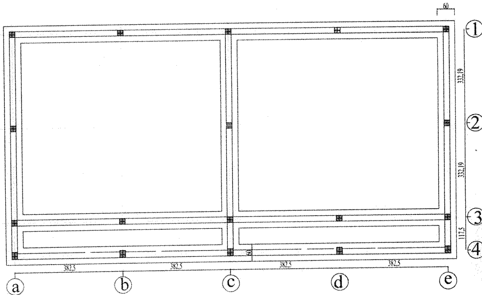
PLAN DE FONDATIONS
